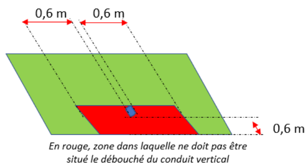
Cas 2 : entrée d'air
