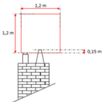
Cas 1 : voisinage d'un conduit de fumée en tirage naturel
