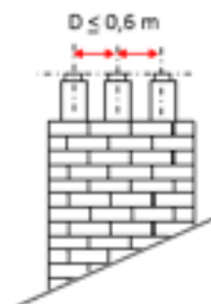
Cas 3 : plusieurs terminaux côte à côte
